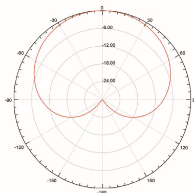
1205MHz-1278MHz
